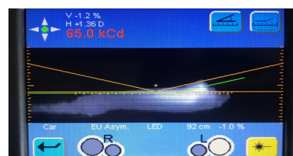
Digitaal koplampafstelapparaat voor het meten van Halogeen, Xenon, bi-Xenon, LED en bi-LED. Dim, groot en mistlampen. incl speciale meetprocedures DLA, Matrix en VLV ILS
