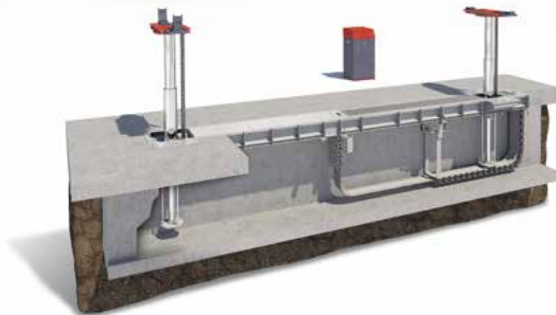
Als frame uitvoering met verzinkt inbouwframe
